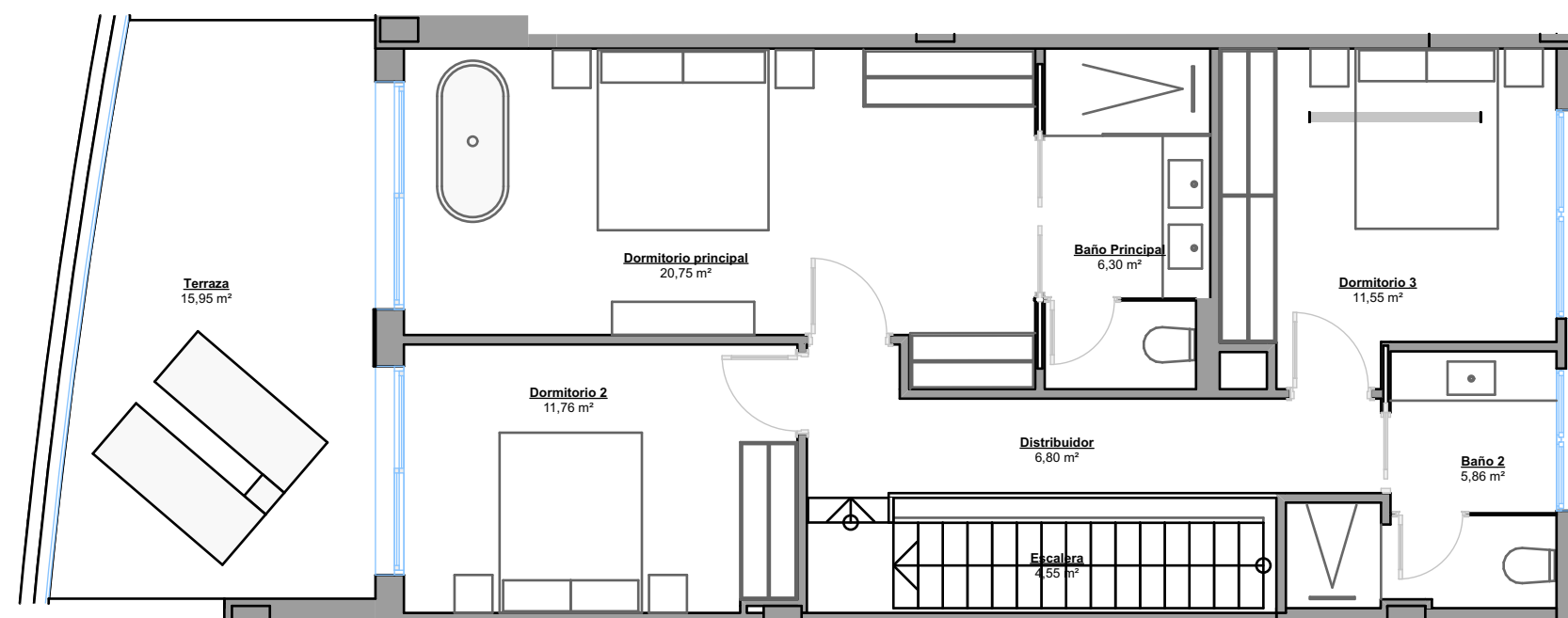
PLANTA PRIMERA
