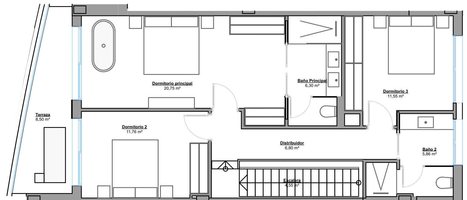
PLANTA PRIMERA
