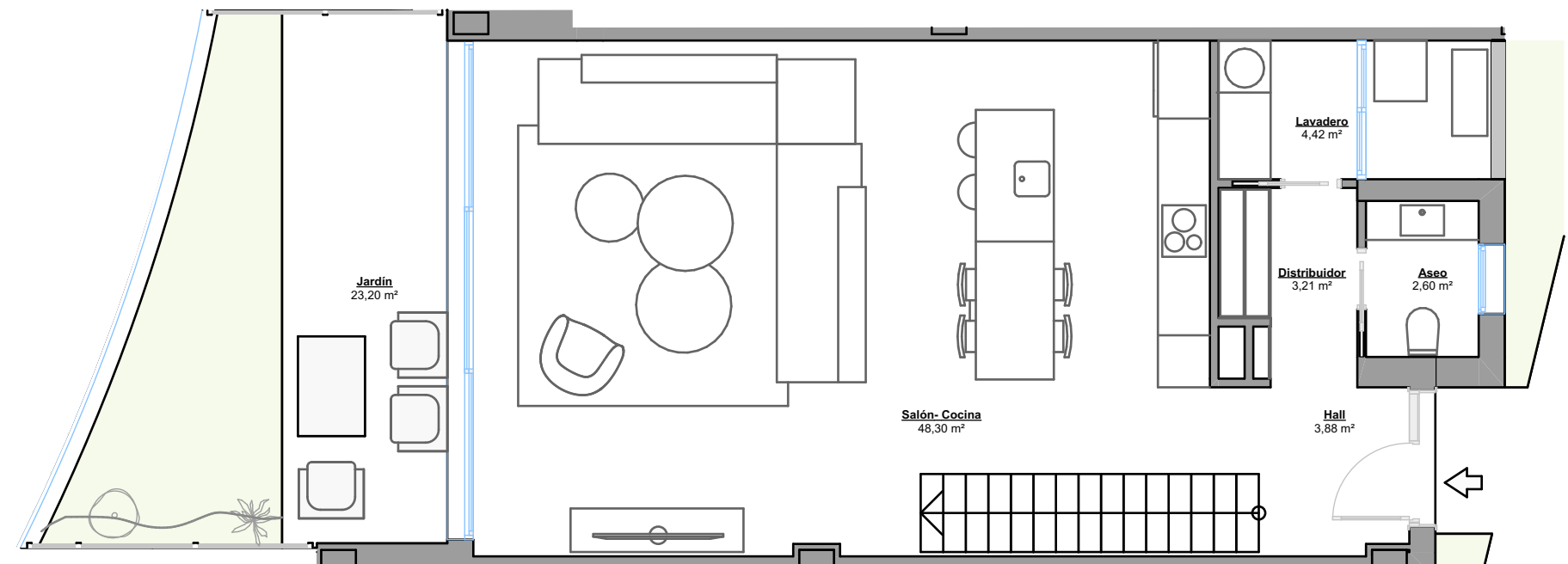
PLANTA BAJA
