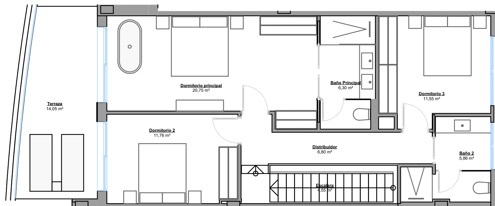
PLANTA PRIMERA
