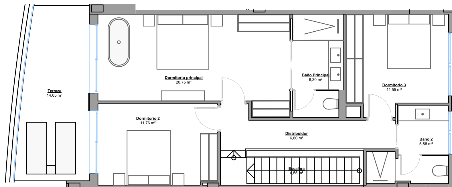
PLANTA PRIMERA
